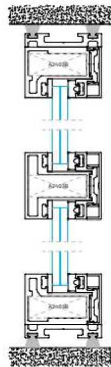
Sección C-C'
