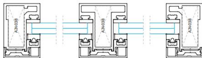
Sección A-A'
