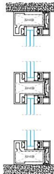
Sección B-B'
