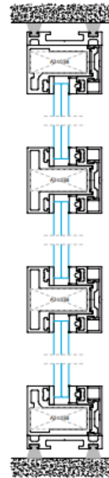
Sección B-B'
