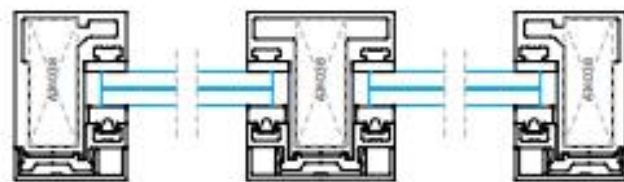
Sección A-A'
