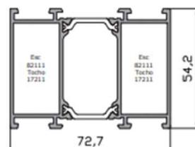
Pilastra puerta. 17473
